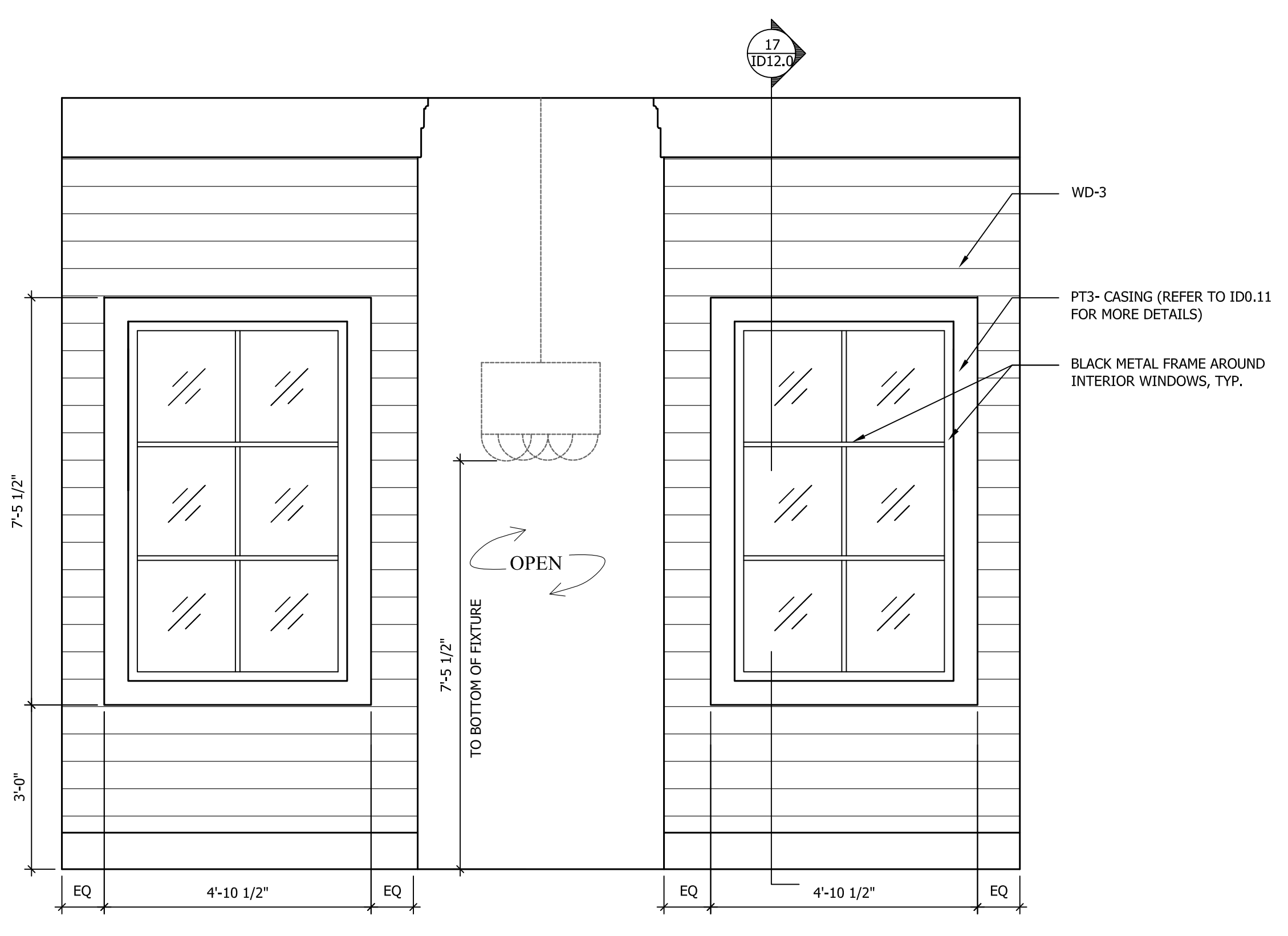
1 LEASING OFFICE ID11.0 SCALE: 1/2" = 1'-0"
