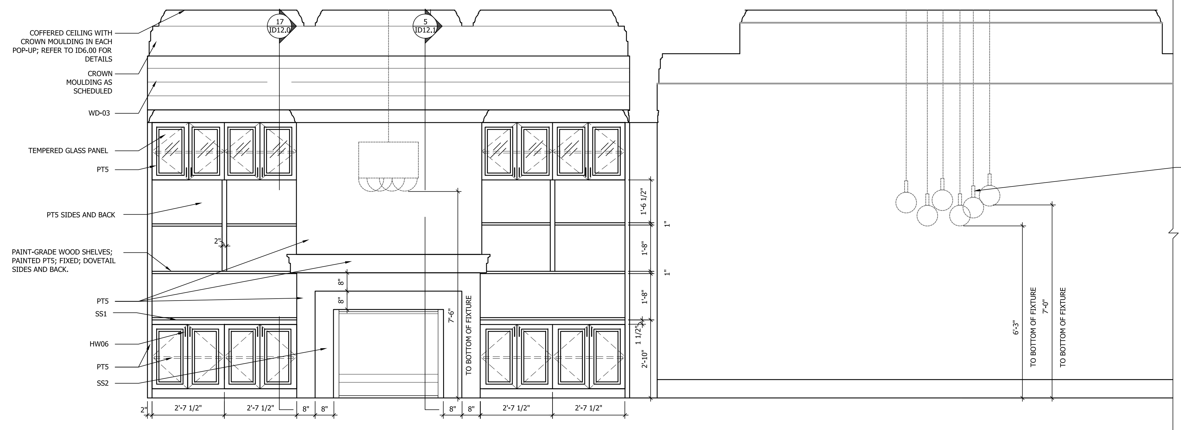
3 WORKROOM ID11.0 SCALE: 1/2" = 1'-0"
