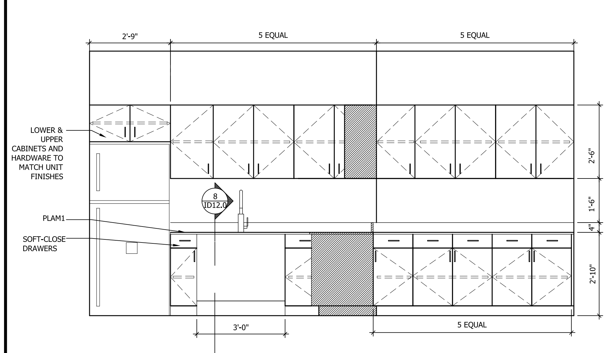
3 WORKROOM ID11.0 SCALE: 1/2" = 1'-0"
