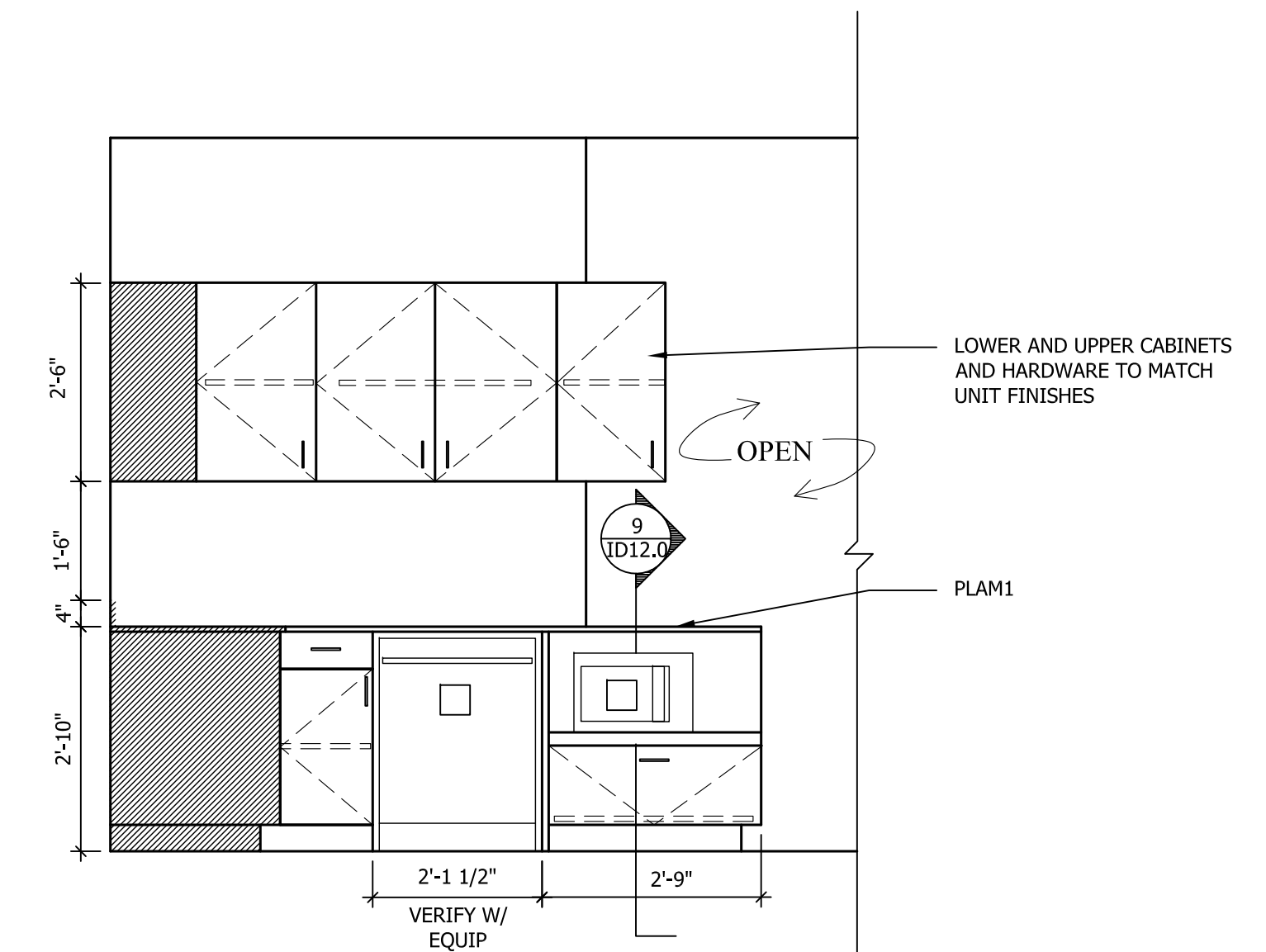
4 WORKROOM ID11.0 SCALE: 1/2" = 1'-0"
