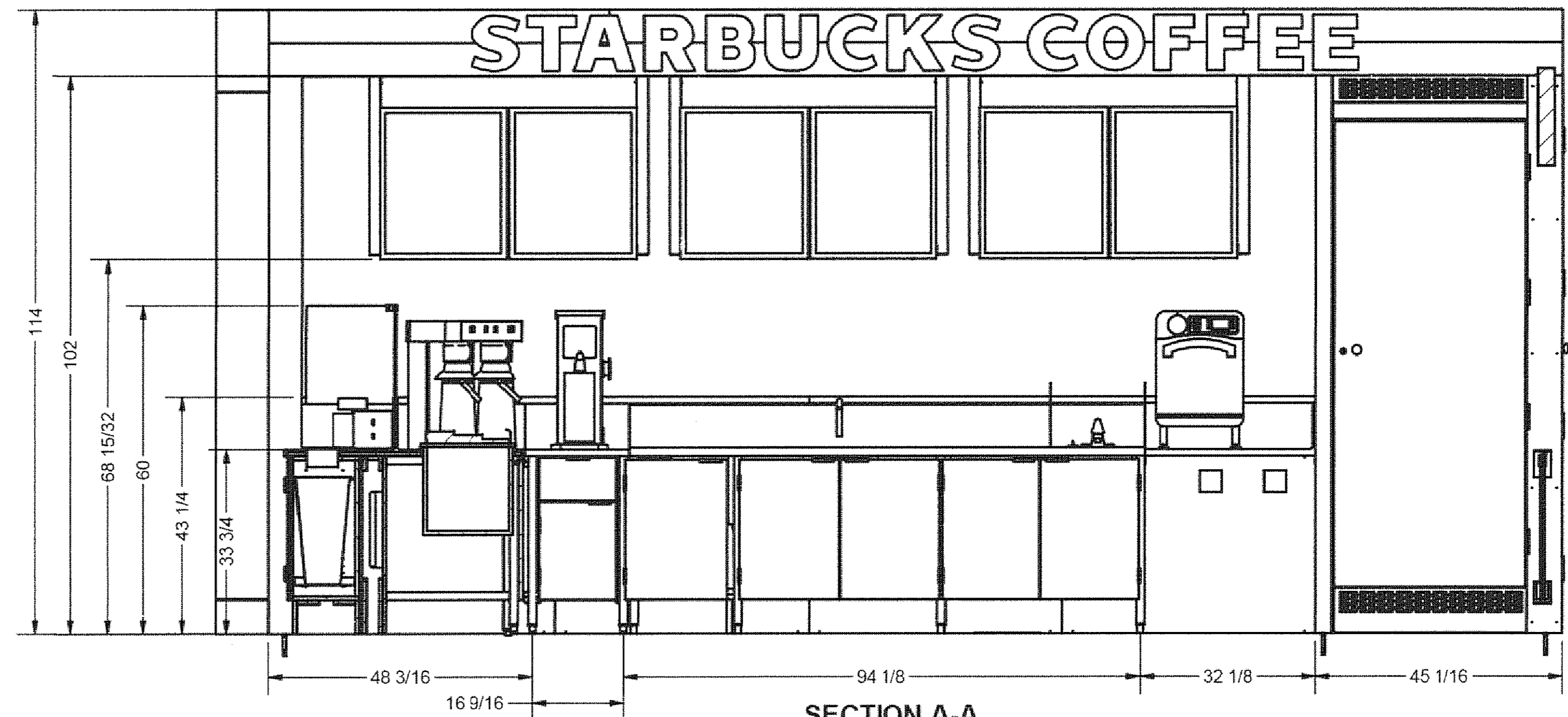
SECTION A-A
